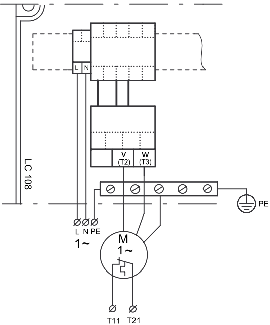
Однофазный электродвигатель
