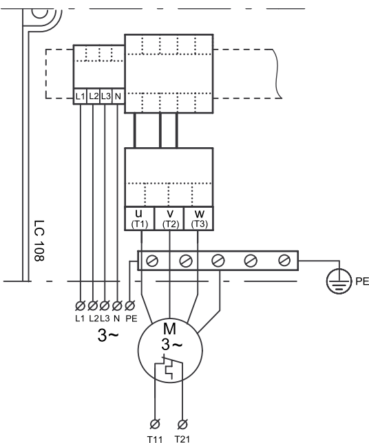
Трёхфазный электродвигатель
