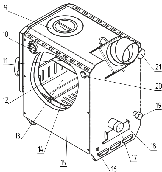
Рис.1 Конструкция отопительного аппарата
