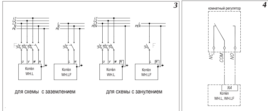
Рис.3 Подключение к электрической проводке
